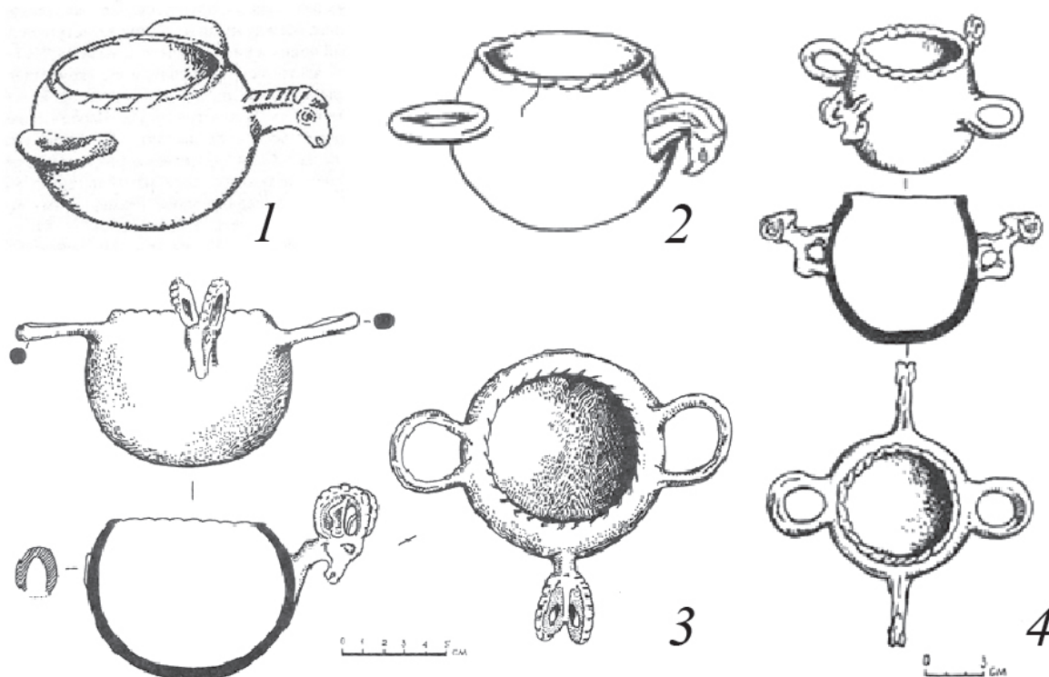
Рис. 3. Медные котелки. 1 – подъемная находка, Имит, долина Ишкоман, Гилгит-Балтистан; 2 – Памир; 3 – могильник Аличур II, курган 2; 4 – Харгуш II, курган 5 (по: Литвинский, 2001, рис. 1–3).
